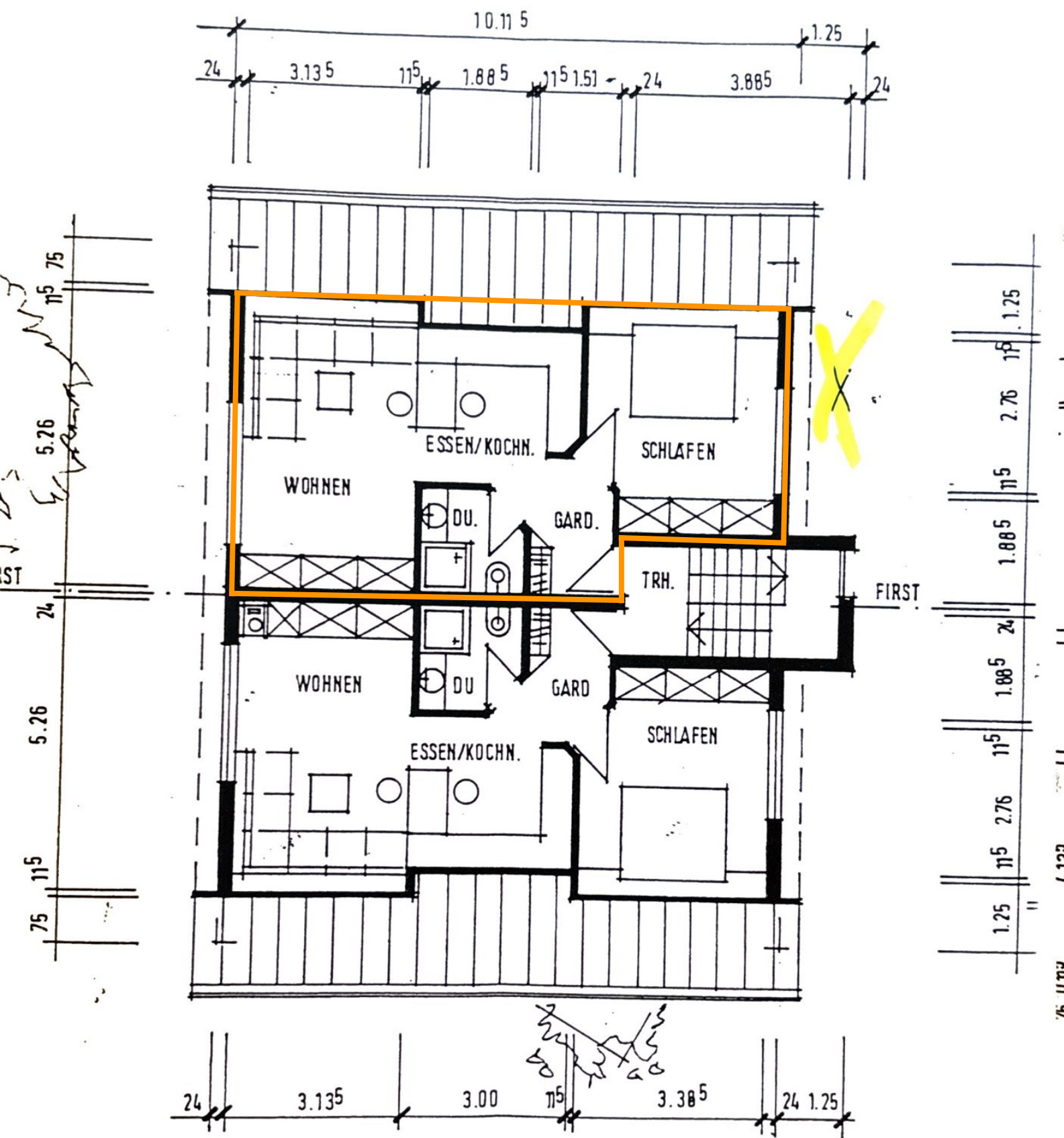
GRUNDRISS DG
